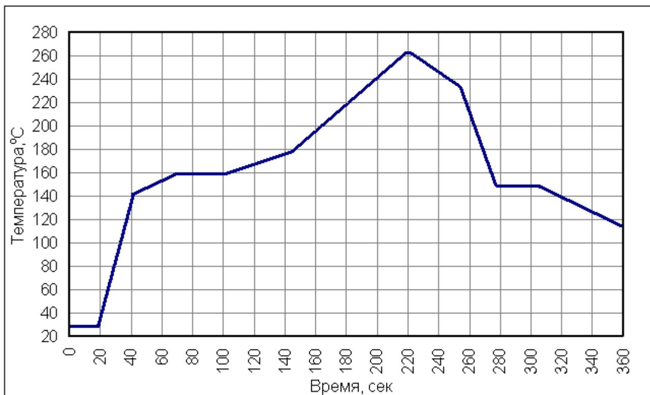
Рисунок 1 - Температурный профиль оплавления при автоматической пайке
